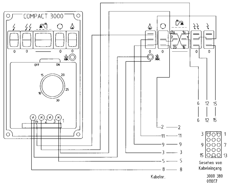
Bedienungstafel, Vorderseite
